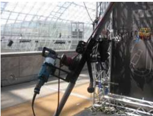
Fig. 9. Cabestano mobile a due velocità, con diverse possibilità di fissaggio. Pensato anche per il rapido recupero . Nell’immagine di sinistra con applicazione di comando motorizzato . PRODUTTORE Skyhook http://www.skyhookrescue.com
