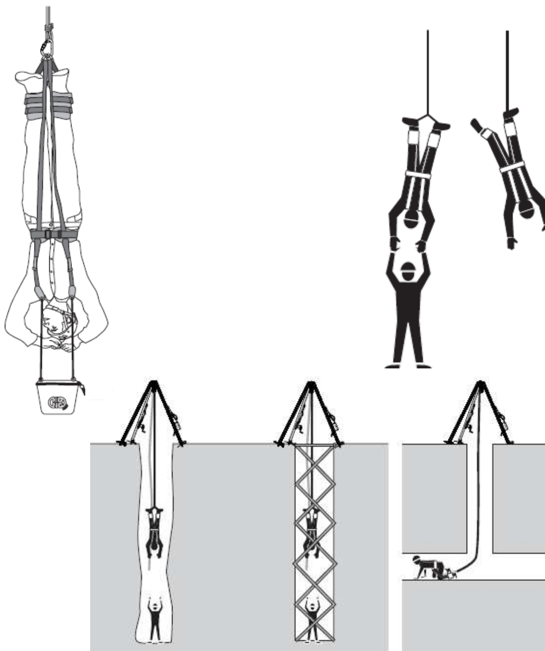
Fig. 15. Cinghia di salvataggio di classe C. Imbracatura di soccorso, con cavagliere conformi alla norma EN 1498 classe C, studiata per la calata di soccorritori in assetto capovolto (a testa in giù). Attenzione questi dispositivi: - sono stati progettati e costruiti esclusivamente per l'utilizzo in operazioni di autosoccorso e/o di soccorso;- devono essere usati da personale ben addestrato e competente. In particolare l'utilizzo dell'imbracatura "Mike" necessita di specifico allenamento nell'operare in assetto ribaltato in quanto la permanenza, anche di pochi minuti, a testa in giù determina cefalee, vertigini, possibili ictus, sensazioni di soffocamento, visione rossa, causate prevalentemente dall'aumento della pressione sanguinea nel cervello. PRODUTTORE KONG modello "Mike": www.kong.it
